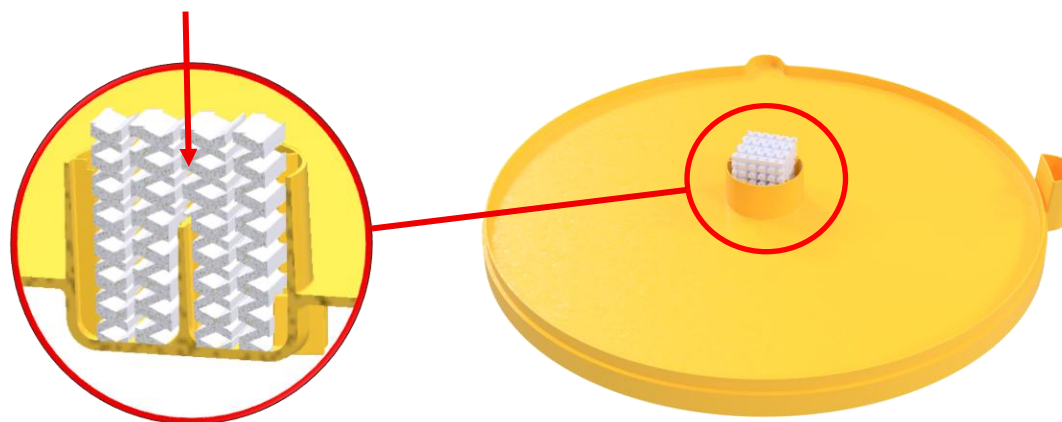
Coupe centrale
