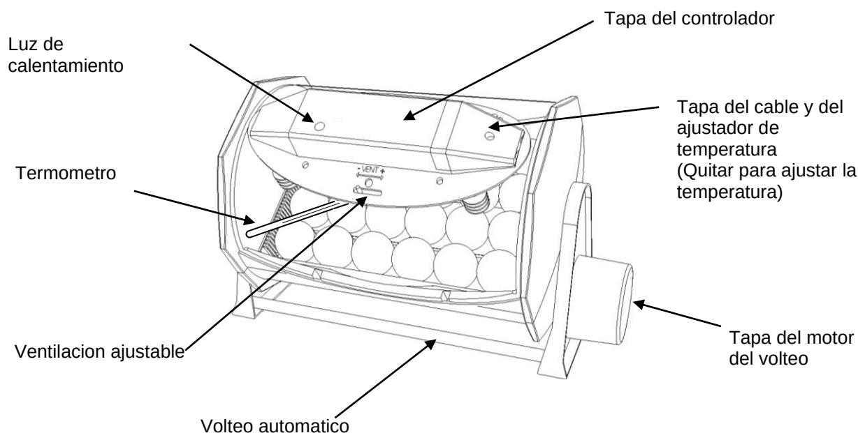
Fig. 1 Características de funcionamiento de la Octagon 20 Eco con volteo automático. (Octagon40 Eco, con funciones similares)
